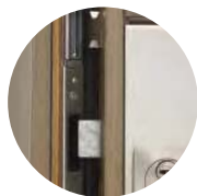
Points de fermeture centraux : - 1 pêne dormant - 1 pêne demi-tour
